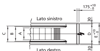
Particolare Y Due o più supporti intermedi
