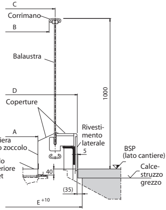
Sezione C-C
