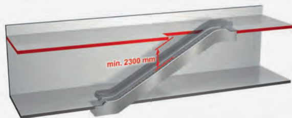
Altezza di passaggio
