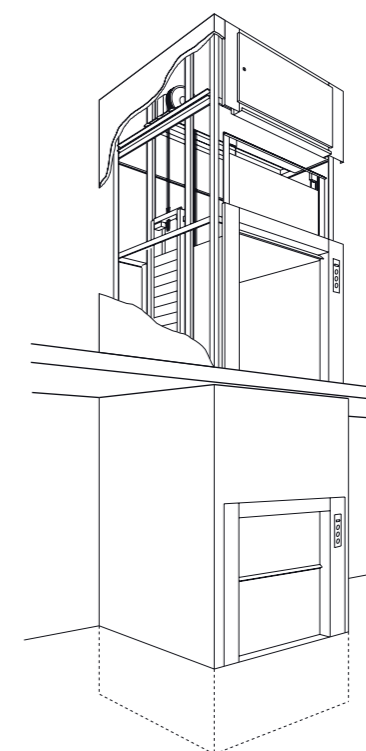
Porte scorrevoli ad altezza del pavimento
